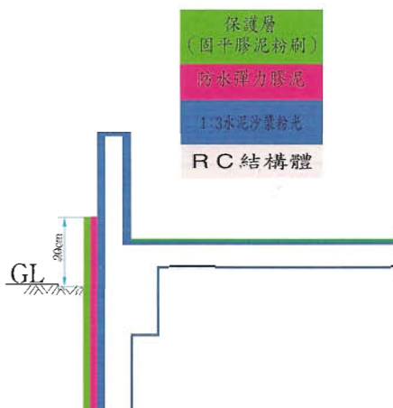
地下室頂收頭處理詳細圖
