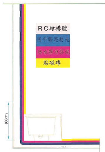
浴廁防水處理詳細圖
