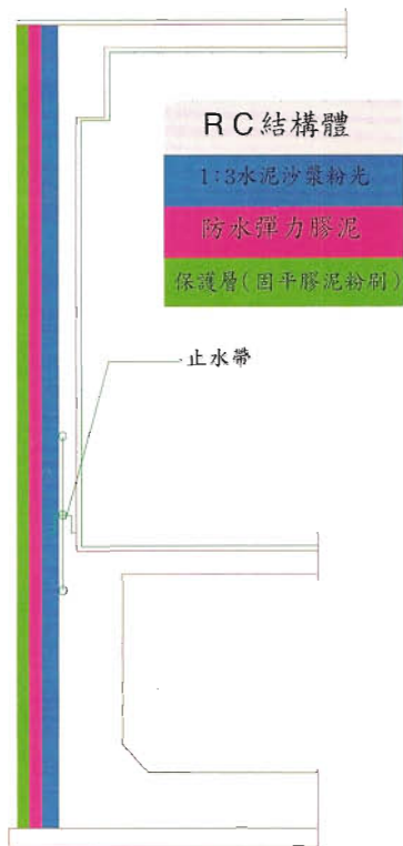
地下室防水處理詳細圖
